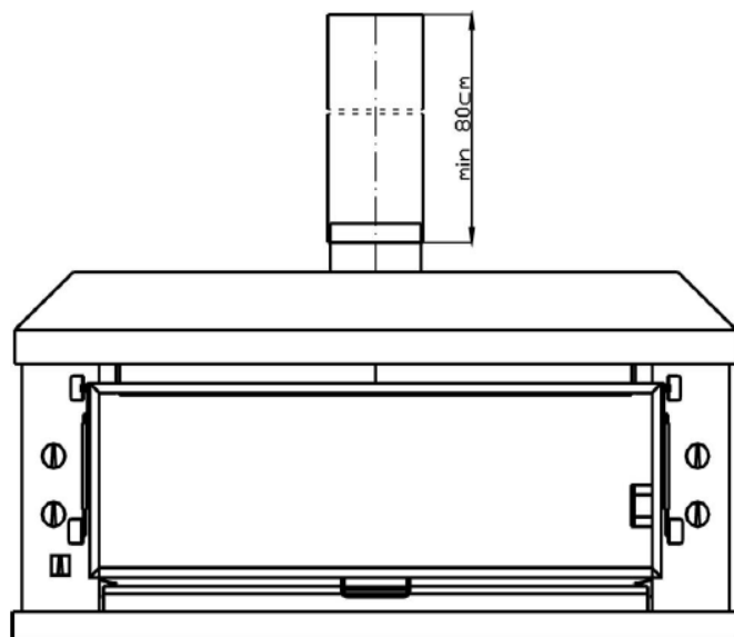
Rys. 5. Sposób podłączenia przedłużenia króćca odprowadzającego spalin
