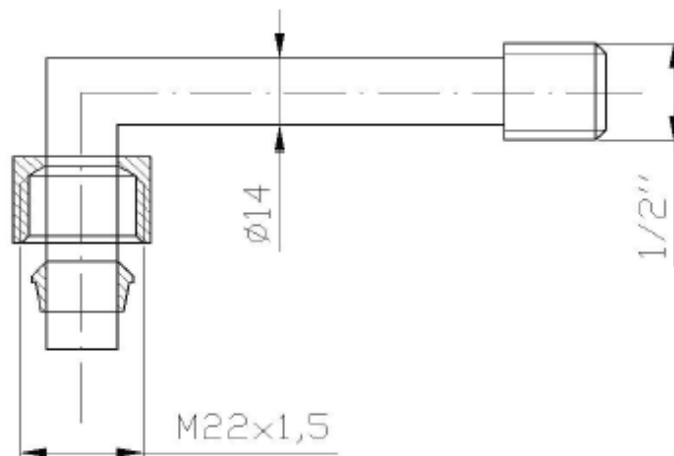
Rys. 3. Króciec przyłączeniowy dla gazu 2E
