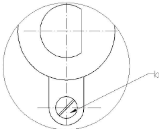
Rys. 6. Widok zaworu gazowego po zdjęciu pokrętła
